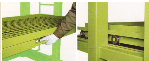
スライド棚 フレーム部分
