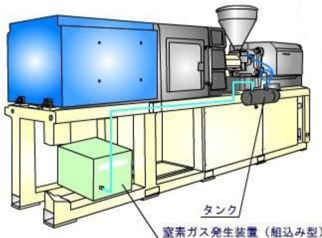
窒素ガス発生装置 (組込み型)
